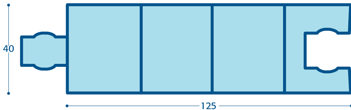
A/1 - PANNELLO PORTA DA 125 x 40 MM.
