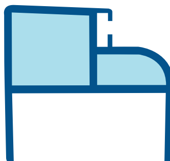
N/10 - PROFILO BATTUTA DOPPIA ANTA NEW
