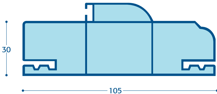
N/2 - PROFILO TELAIO NEW DA 105
