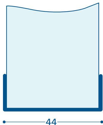
N/9 - GUIDA SOTTO
