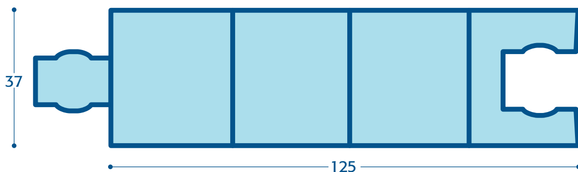
A/37 - PANNELLO PORTA DA 125 x 37 MM. IN PVC RIGENERATO
