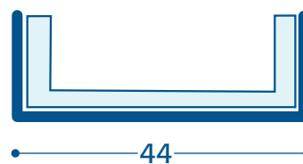
N/9 - GUIDA SOTTO CON RINFORZO
