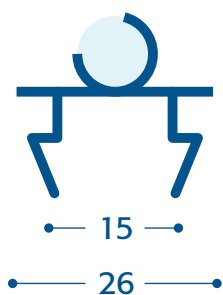
ART. 45 PROFILATO A SCATTO PARTENZA
