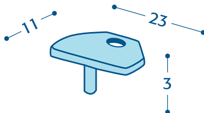
ART. E/F PIASTRINA IN PVC PER FINESTRATO
