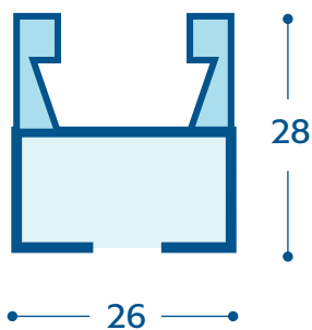
ART. 44 GUIDA DI SCORRIMENTO E ATTACCHI LATERALI
